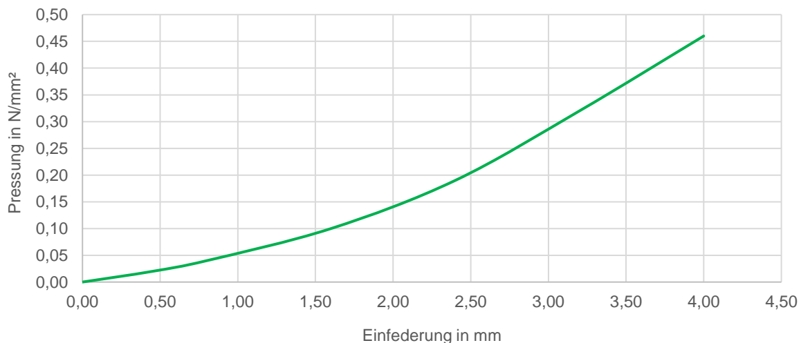
Einfederung
