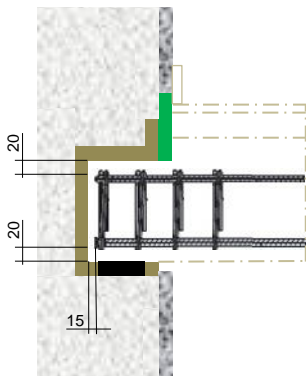
Vertikalschnitt:
